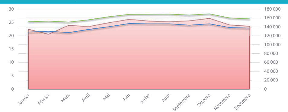
9 Consommation mensuelle d'électricité et les températures moyennes diurnes et nocturnes au Raizet, en 2015
