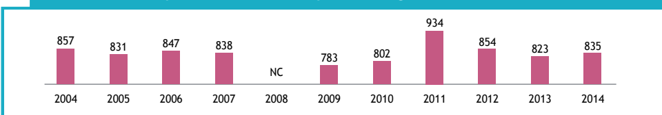
44 Émissions CO 2 de la production d'électricité par KWh (en gramme)
